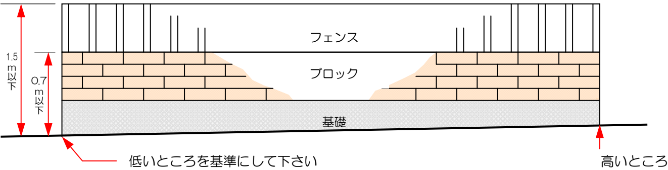
3-2 道路側から見たへの設置例
