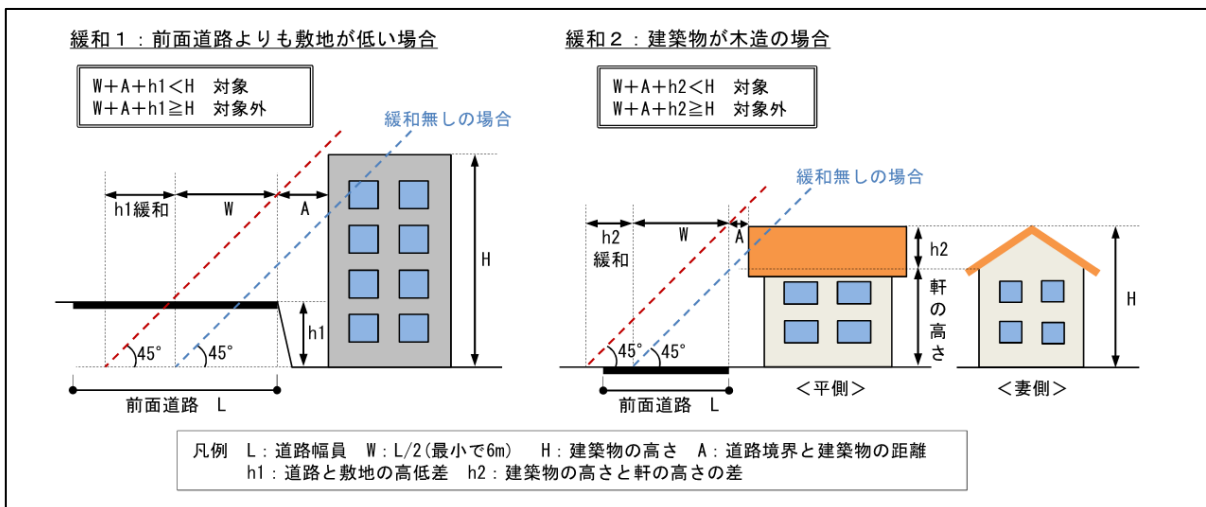
図 2-2 通行障害建築物の緩和の要件
