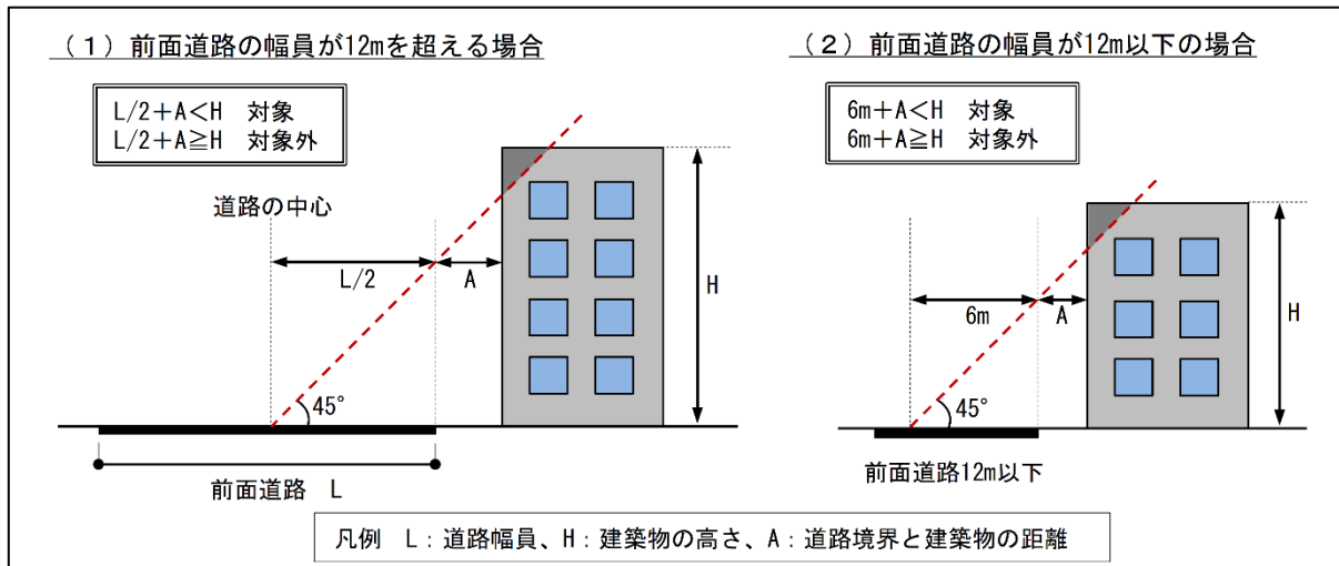
図 6-2 通行障害建築物の対象となる要件
