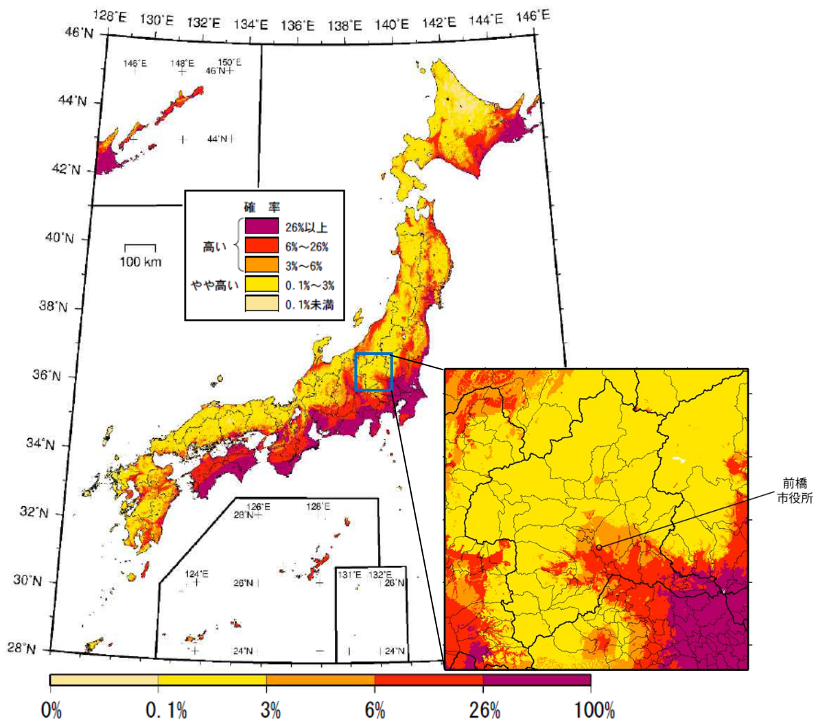
図 3-2 全国地震動予測地図 2020 年版
