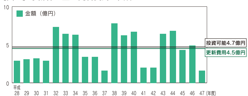
【図4】予防保全型の更新費用の試算
